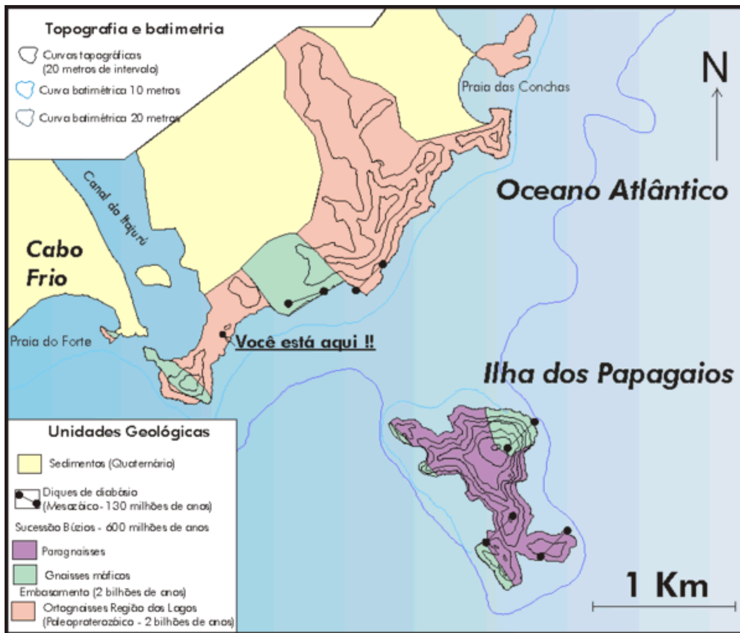
Figura 2 - Mapa geológico da área do Parque da Boca da Barra e Ilha dos Papagaios.
